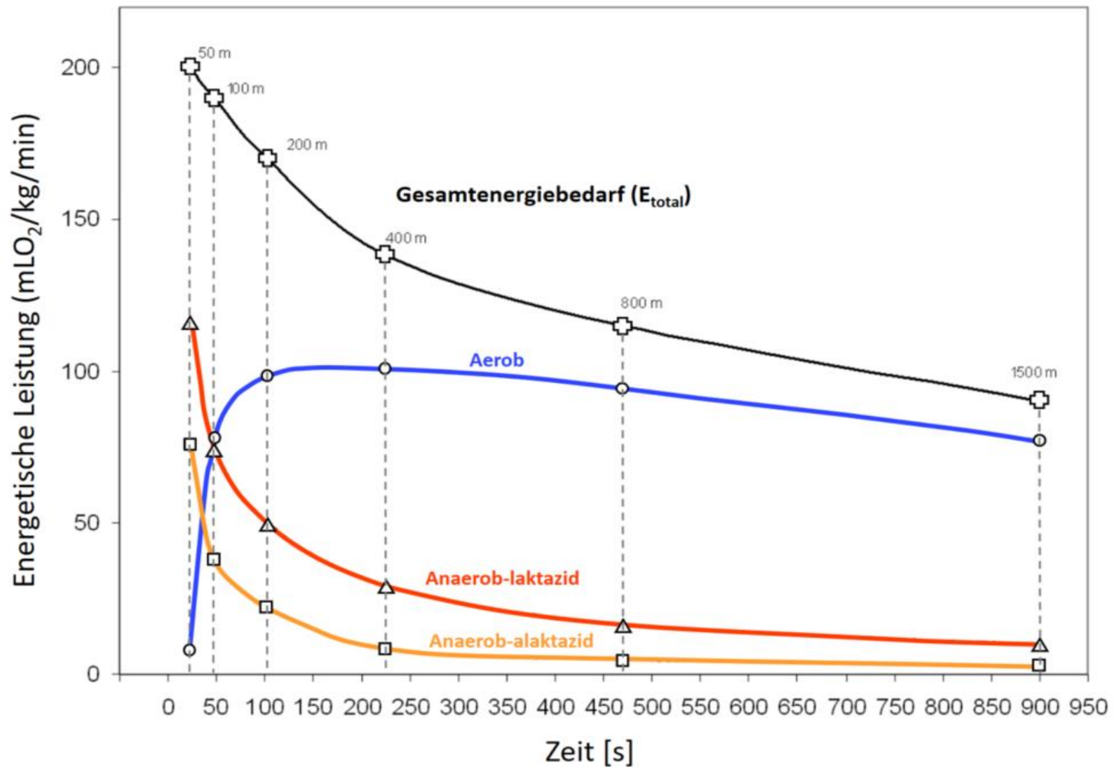
Abb. 2. Gesamtenergiebedarf sowie die Anteile der einzelnen energieliefernden Systeme für die Schwimmdisziplinen von 50m bis 1500m (mod. nach Rodriguez & Mader. Energy systems in Swimming. In Seifert, Chollet und Mujika. (2011). World Book of Swimming)
